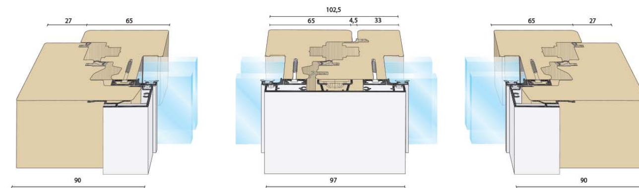
SEZIONE ORIZZONTALE INFISSO A 2 ANTE
