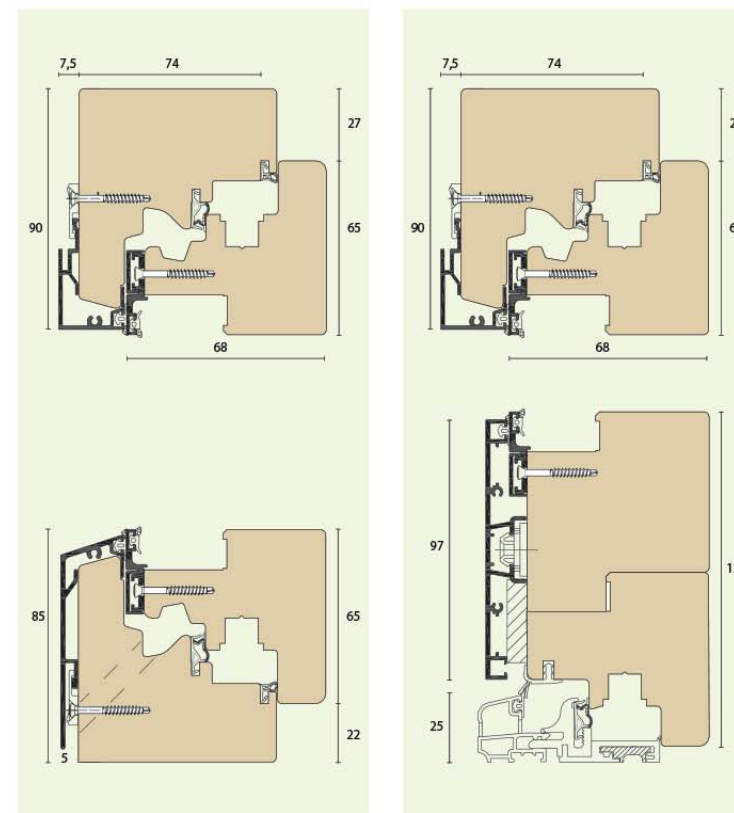
SEZIONE VERTICALE FINESTRA
